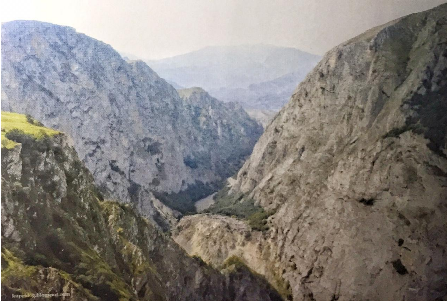
Şəkil 5. Qaraçay kanyonu. Panorama. Cənubdan görünüş.
