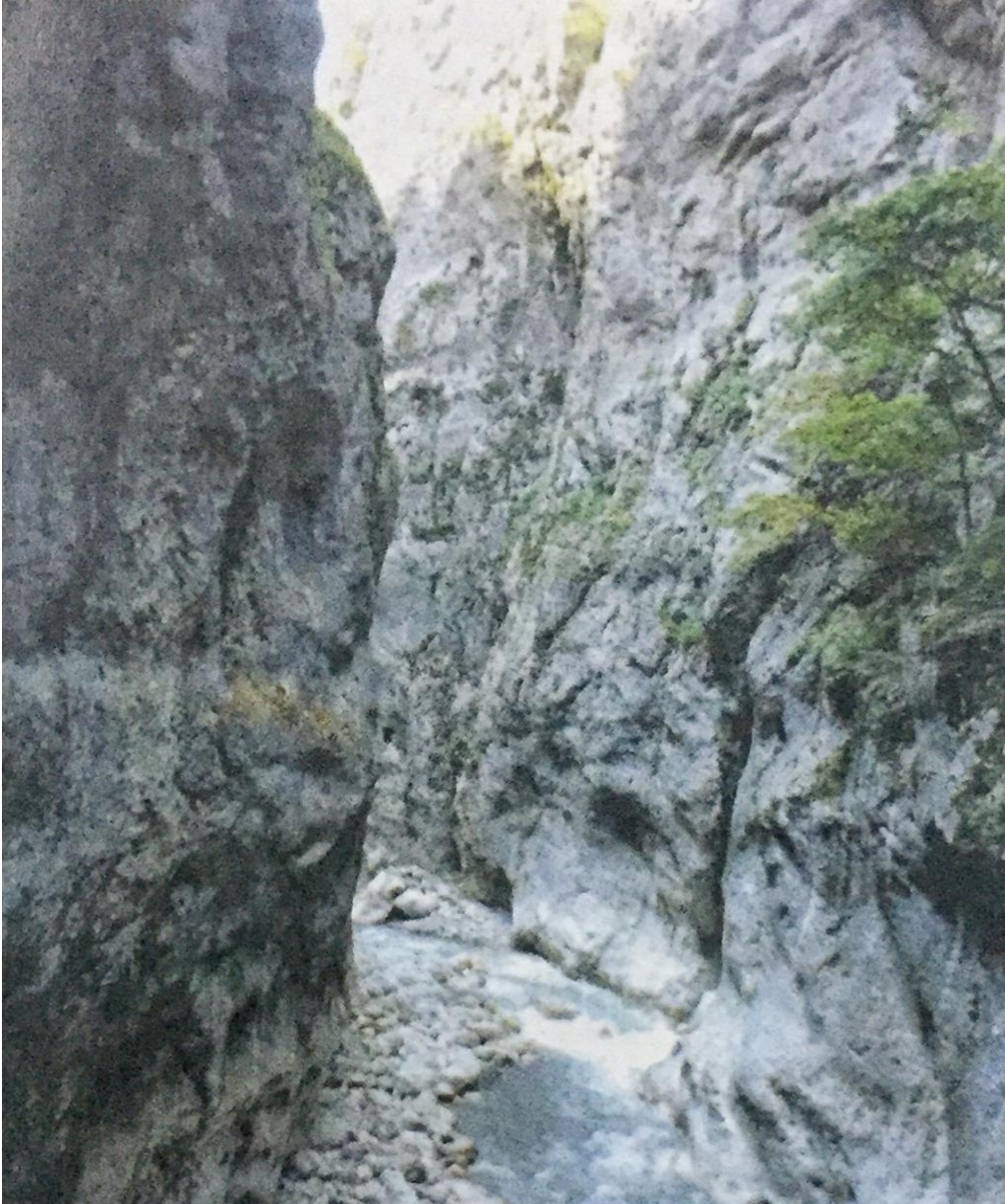
Şəkil 6. Zəngiçay kanyonu.
